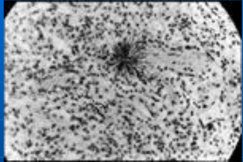
Partículas alfa liberadas por un polvo de plutonio de una micra dentro de un tejido pulmonar.
